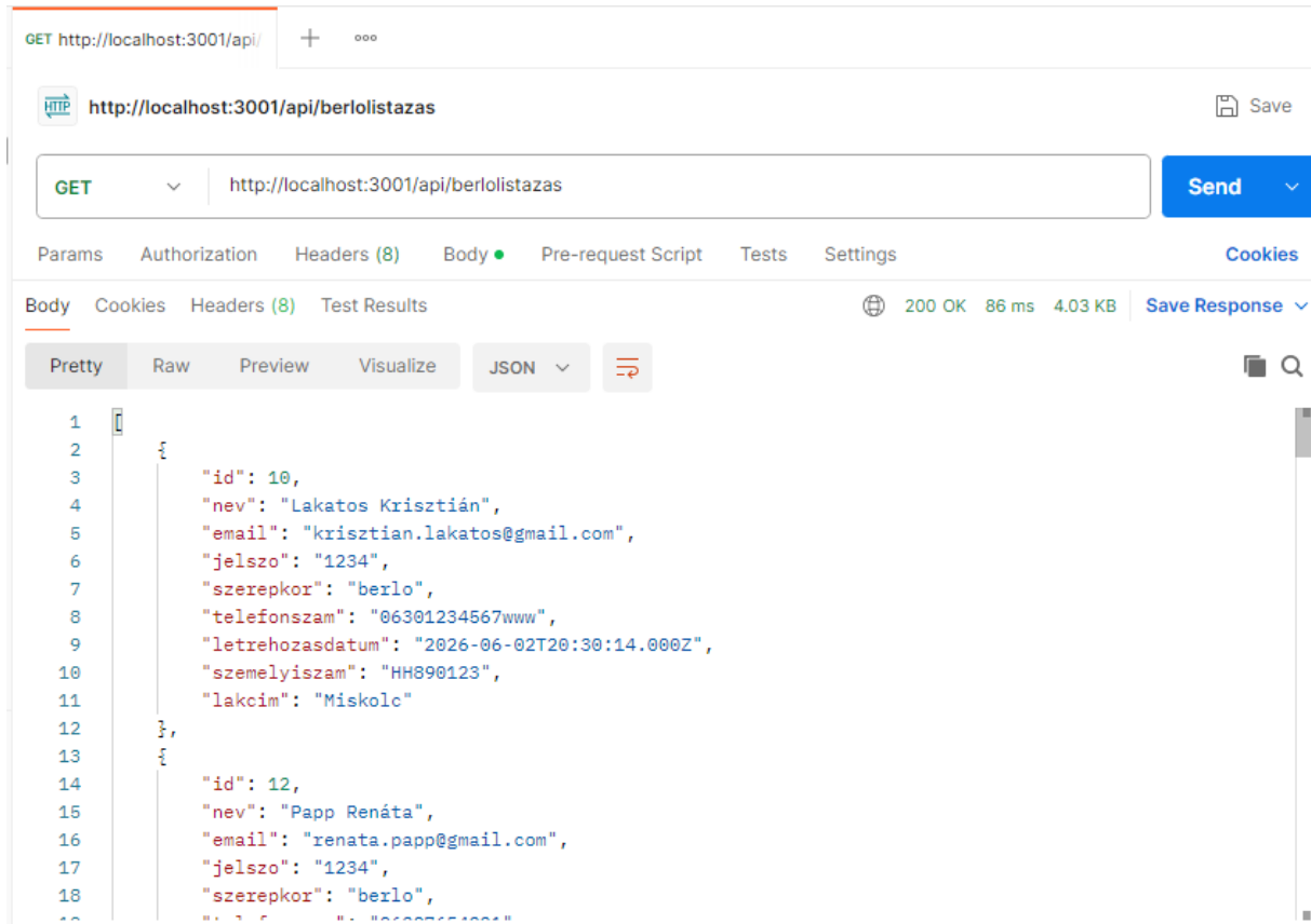
1.Kép: Bérlők listázásának Postman tesztelése.
